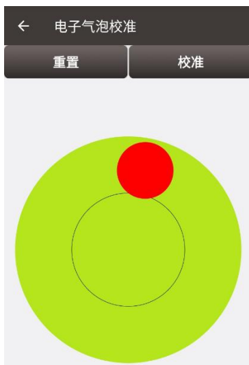
图 2.9 调节前的电子气泡
