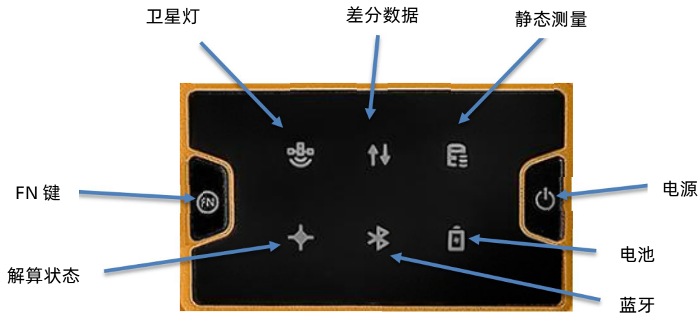
图 1.6 基础版的按键和 LED 灯
