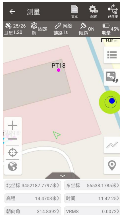
图 4.20 倾斜补偿状态已开启
